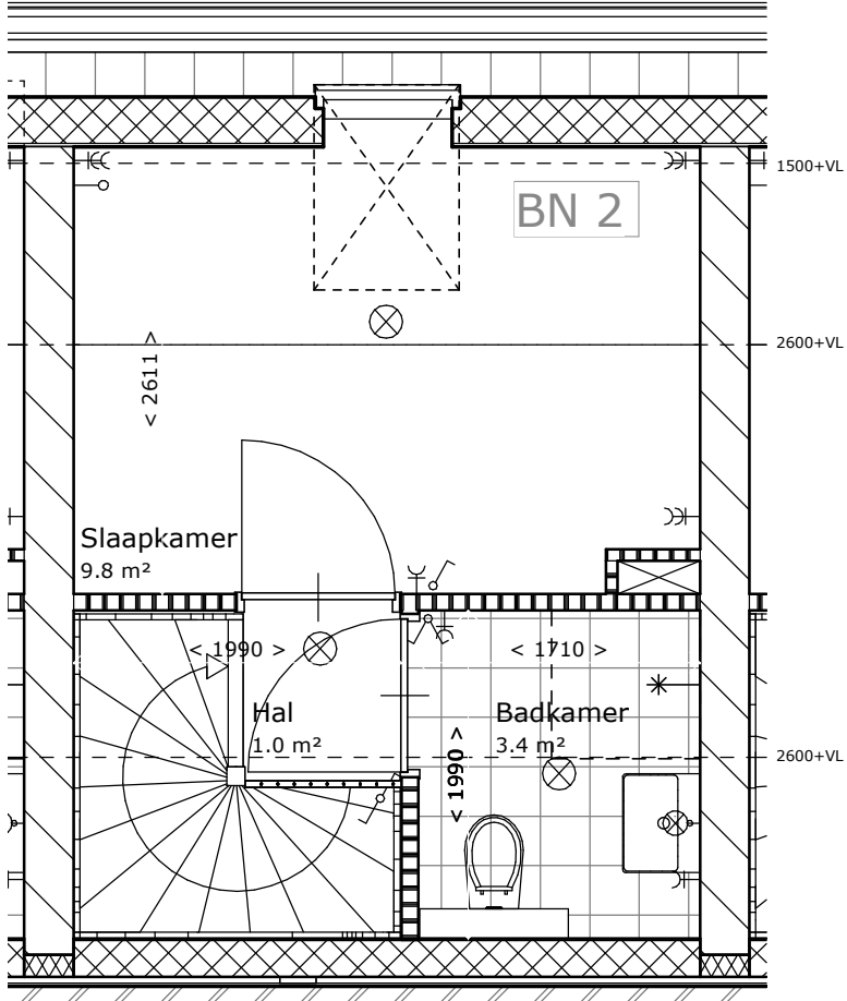
Tweede verdieping
