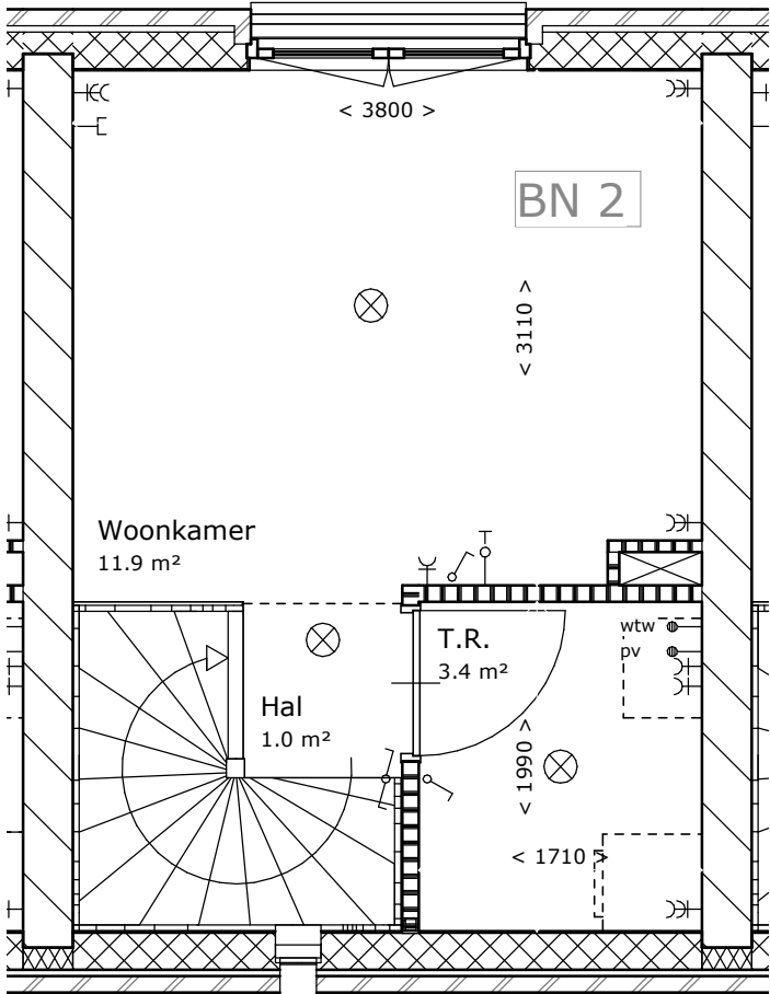
eerste verdieping
