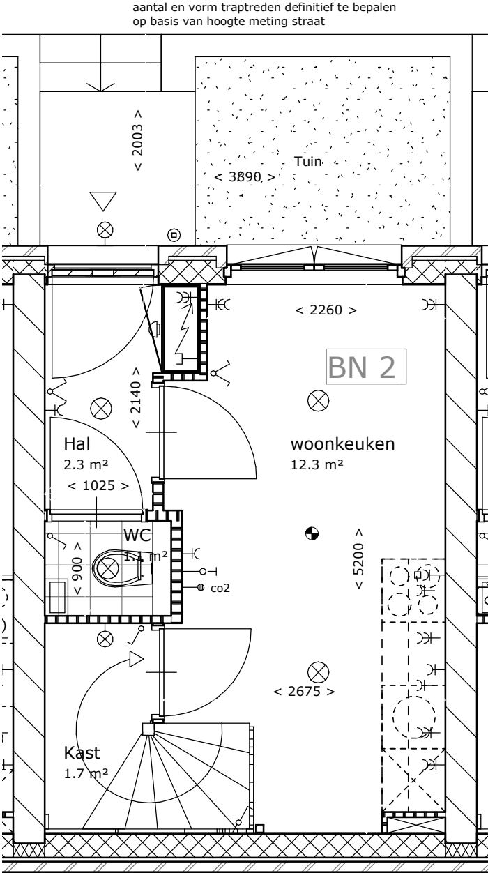
begane grond
